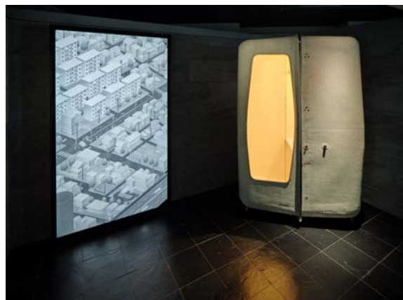
1964年に日ポリ化工によって製作され、戦後の住宅における入浴習慣を大きく変えた日本初の洗い場付きオールFRP製カプセルユニットバス。会社の歴史上、2番目に制作されたもので通称『2号機』。
